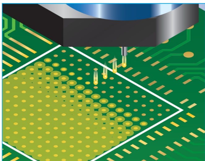
助焊剂点胶
